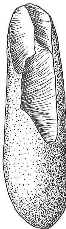
Chopping Tools - Littoral de PLŒMEUR-56 A- Galet de Quartzite. B- Galet de Quartz. dessins Marc GALLUDEC
